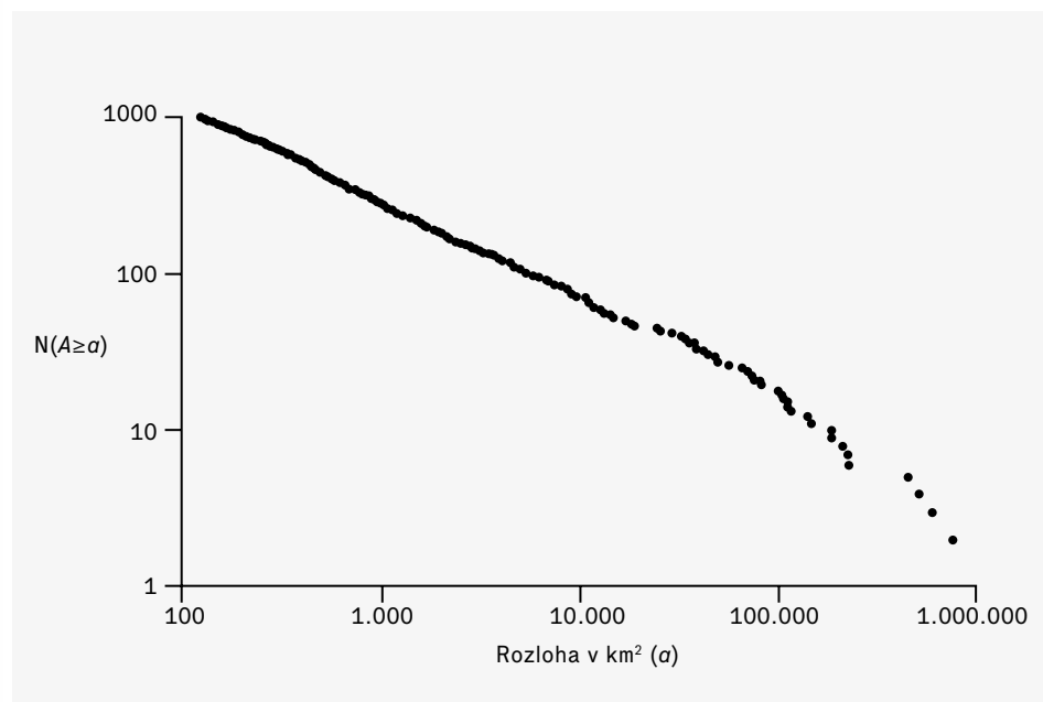
OBR. 10 – Log-log graf velikostní diferenciace ostrovů světa (ostrovy větší než 100 km 2 ); pozn.: jedná se o soubor 1.073 ostrovů, kde na ose y je zachycen počet ostrovů (N) s rozlohou, která je větší či rovna určité rozloze, zdroj: Novotný (2010)
